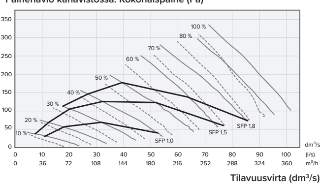
Painehäviö kanavistossa. Kokonaispaino (Pa)
